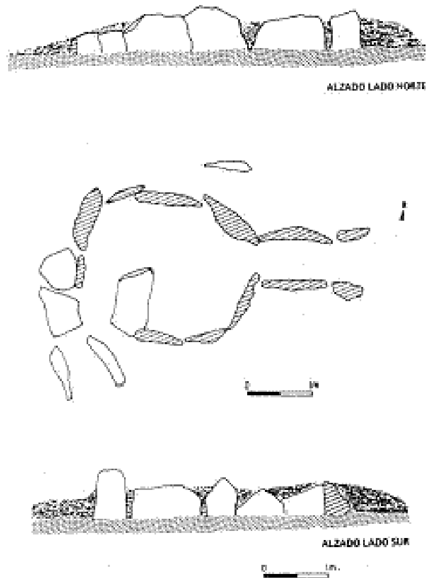
Fig. 13.- Planta y alzado de la sepultura 3.
